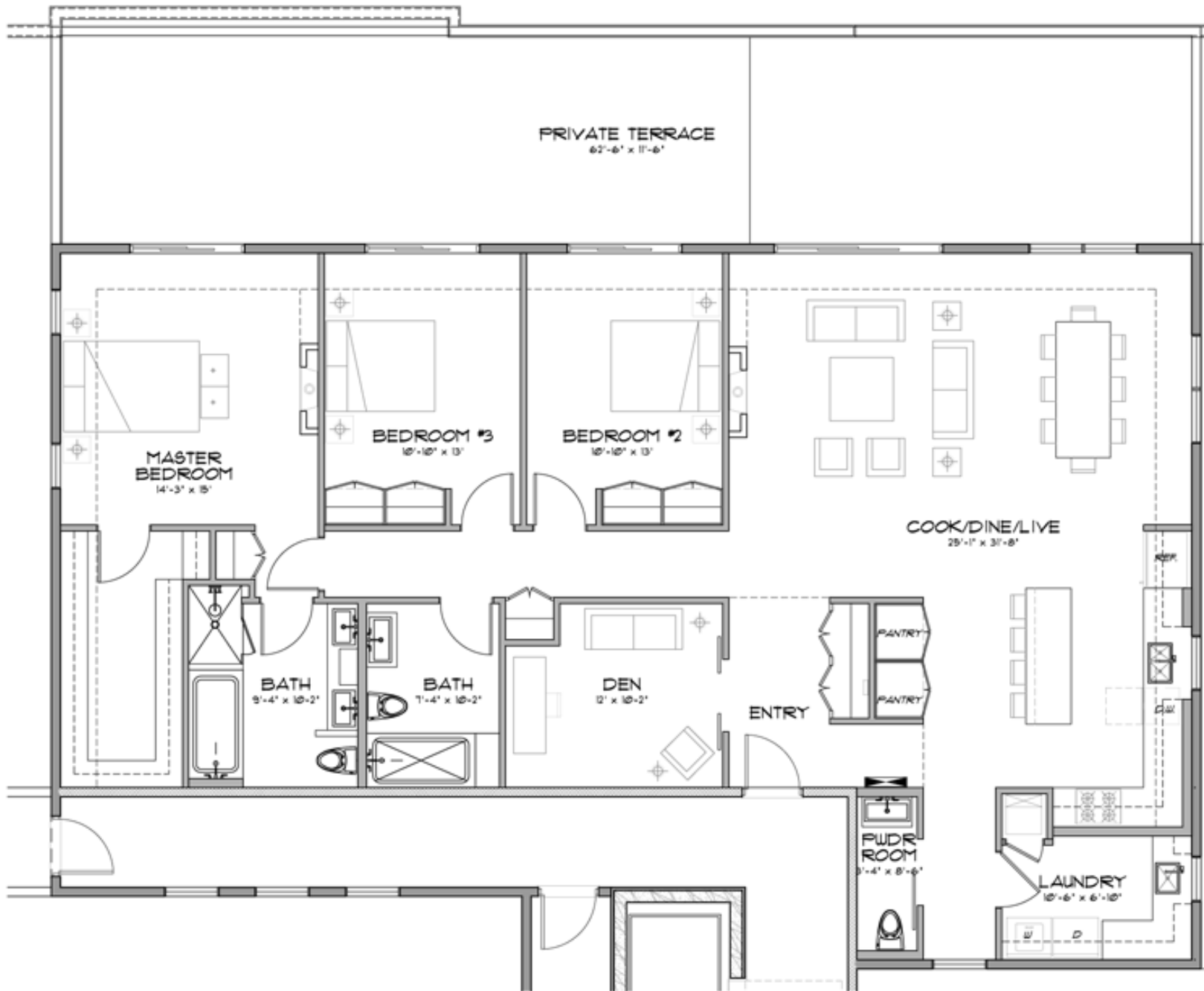
UNIT TYPE E1 - 2,020 S.F.
